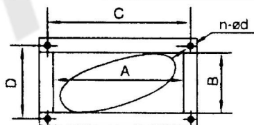
新风进口法兰外形尺寸安装示意图
