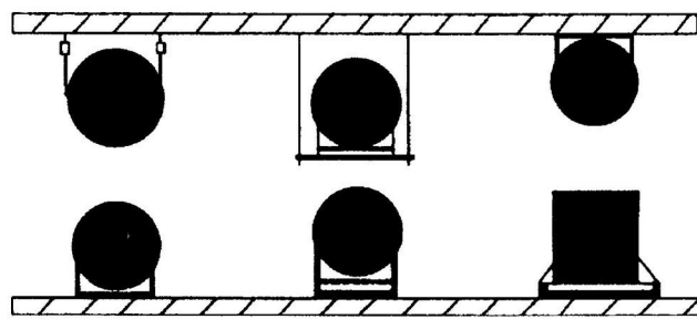
HL3-2A 型风机工程安装建议图
