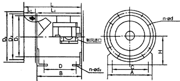
PYHL-14A 型风机外形安装尺寸示意图
