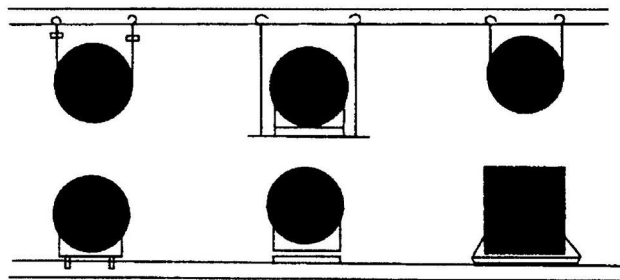
PYHL-14A 型风机工程安装建议图
