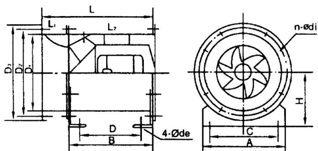
HL3-2A 型风机外形安装尺寸示意图
